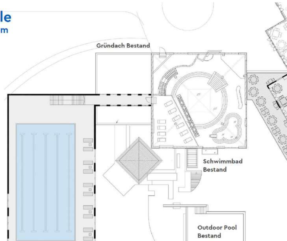
Grundriss EG Neubau Schwimmhalle
